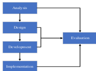
Gambar 3. Tahapan ADDIE
