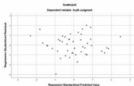
Sumber : Output SPSS Versi 25 Gambar 2. Uji Heteroskedasitas
