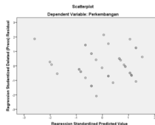
Gambar 2. Uji Heteroskedastisitas
