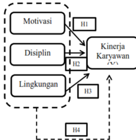
Gambar 1. Kerangka Konseptual
