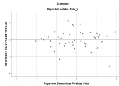
Gambar 2 Scatterplot Heterokedastisitas
