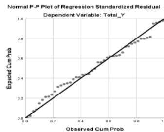
Gambar 3. Uji Normalitas
