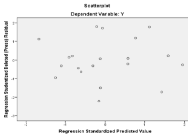
Gambar 2. Uji Heteroskedastisitas
