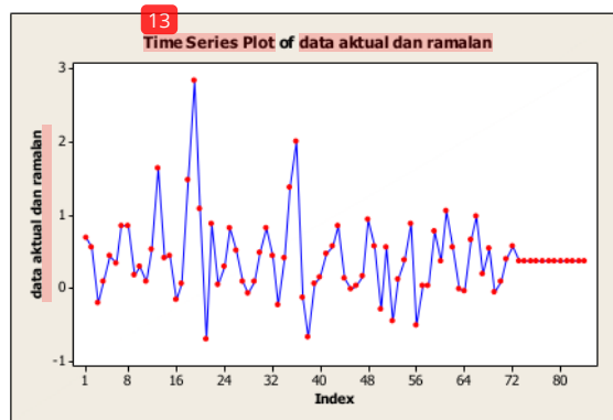
Gambar 2. Plot Time Series Gabungan Data Aktual dan Ramalan
